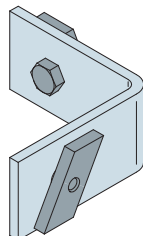
② Angle de plinthe avec raboutage
