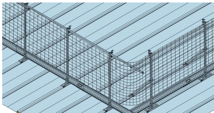
CAVALIER BAS DE PENTE MLFFP03/01
