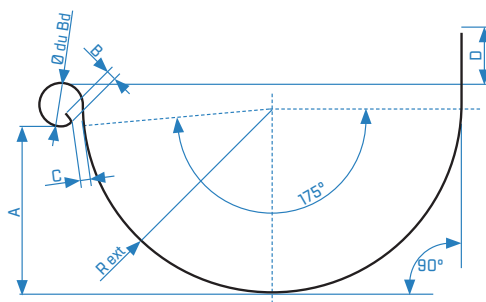
CARACTÉRISTIQUES 1/2 LUNE
