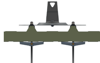
FIXATION PAR CHEVILLE À BASCULE SUR PANEAU SANDWICH
