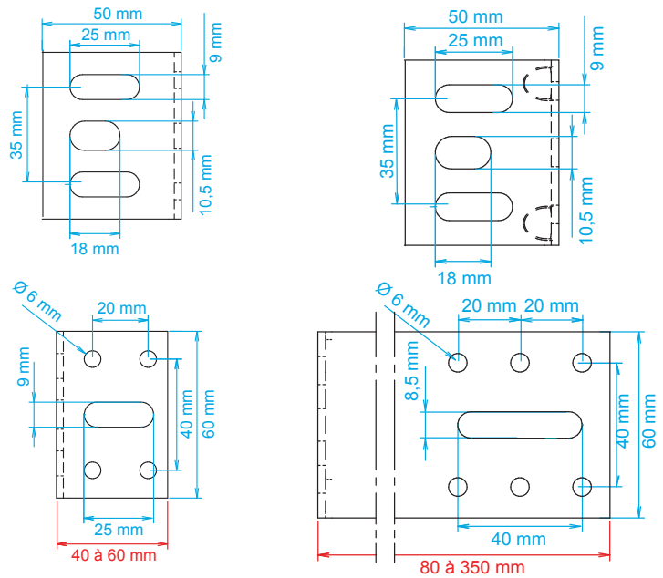
La longueur des équerres varie en fonction de l'épaisseur de l'isolation
