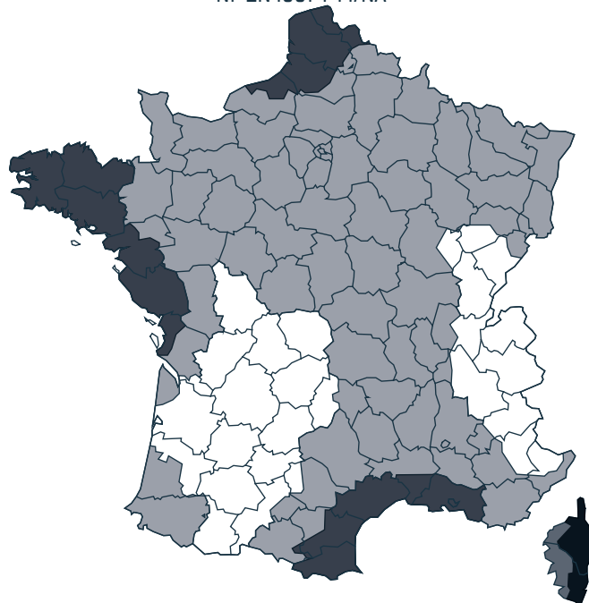
Carte de la valeur de base de la vitesse de référence en France NF EN 1991-1-1-4/NA:2008-03 NF EN 1991-1-14/NA
