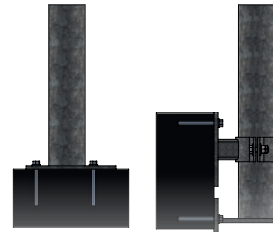
FIXATION PAR CHEVILLE À BASCULE SUR PANEAU SANDWICH
