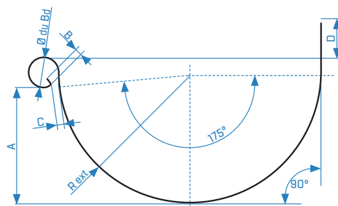
CARACTÉRISTIQUES 1/2 LUNE
