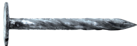
Ø tête : 13 mm 3.5 x diamètre de la tige
