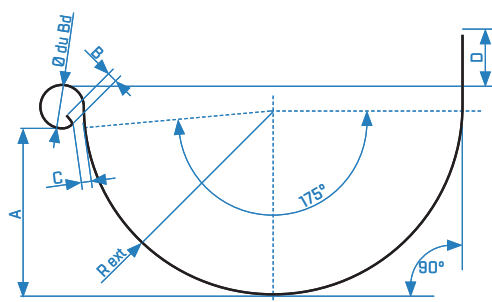
CARACTÉRISTIQUES 1/2 LUNE
