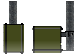
FIXATION PAR ANCRAGE CHIMIQUE (PAR LE DESSUS / LATÉRAL)
