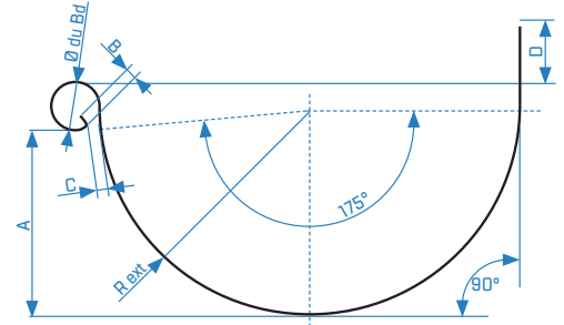
CARACTÉRISTIQUES 1/2 LUNE
