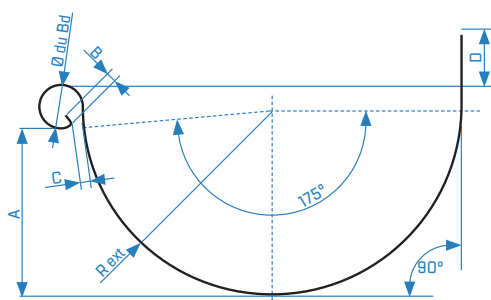
CARACTÉRISTIQUES 1/2 LUNE
