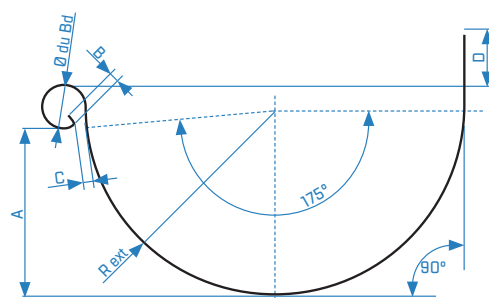
CARACTÉRISTIQUES 1/2 LUNE
